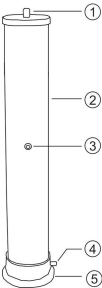
带抽头款 ①高压端 ②绝缘筒 ③中间抽头 ④接地端 ⑤底座
